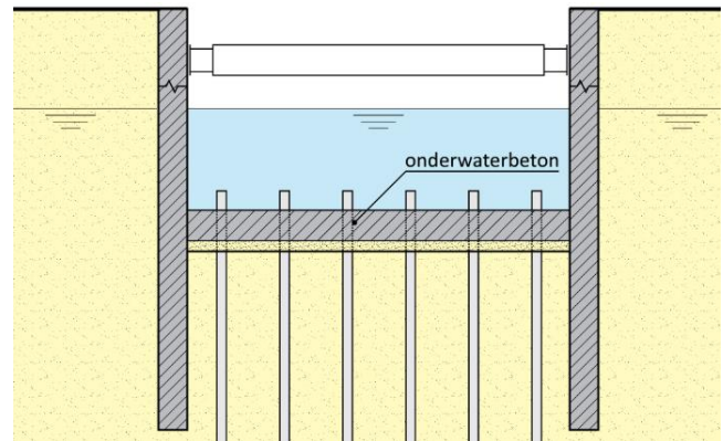
Afbeelding 2: principedoorsnede van de bouwkuip met onderwaterbeton.
