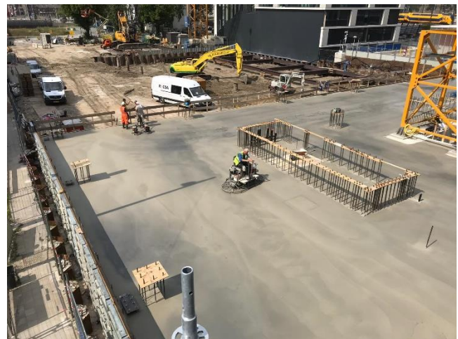
Afbeelding 6: Het vlianderen (vlak maken) van de betonvloer.
