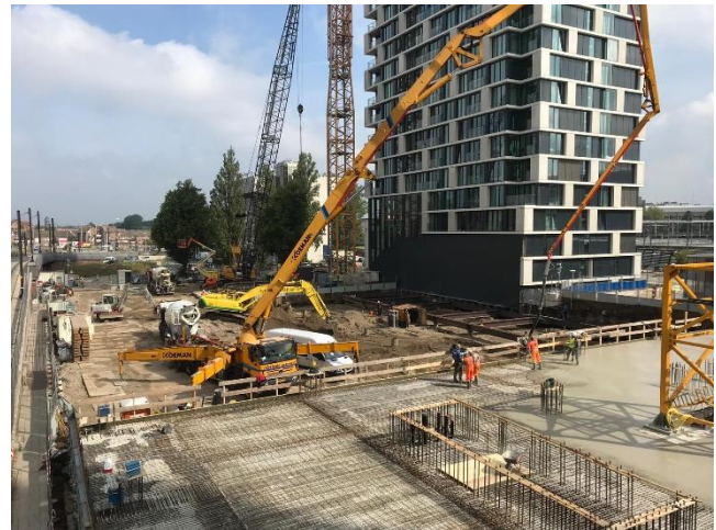
Afbeelding 5: Het storten van de betonvloer.
