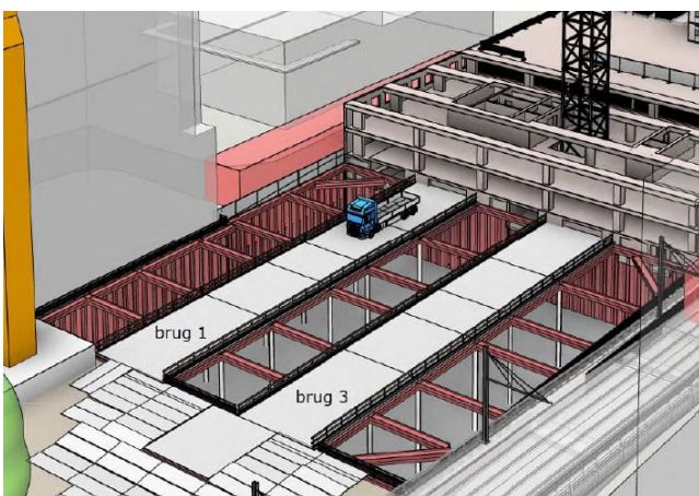
Afbeelding 4: De voorbereidingen voor brug 1 worden getroffen.
